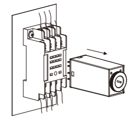
(4) 拔出继电器
