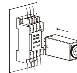
(3) 装上继电器
