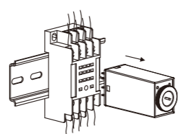
(10) 拔出继电器
