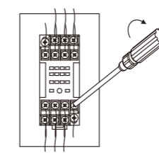
(2) 按底座顺序号接上导线并拧紧接线螺钉
