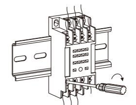
(8) 按底座顺序号接上导线并拧紧接线螺钉
