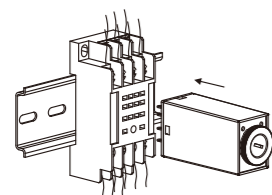
(9) 装上继电器
