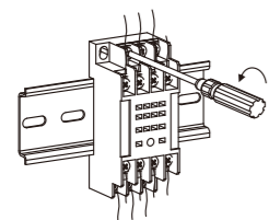
(11) 拧松接线螺钉并拆除导线
