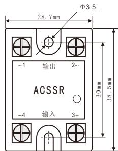
安装尺寸（单位mm）
