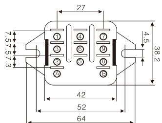
顶部(B)型法兰式尺寸图
