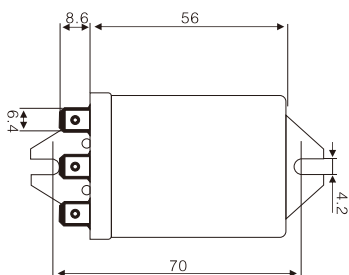
顶部(B)型法兰式尺寸图
