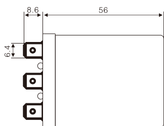
小基座尺寸图
