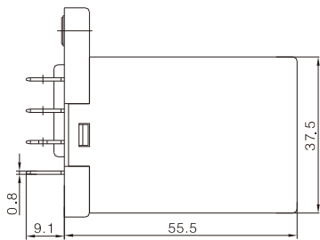
小基座尺寸图
